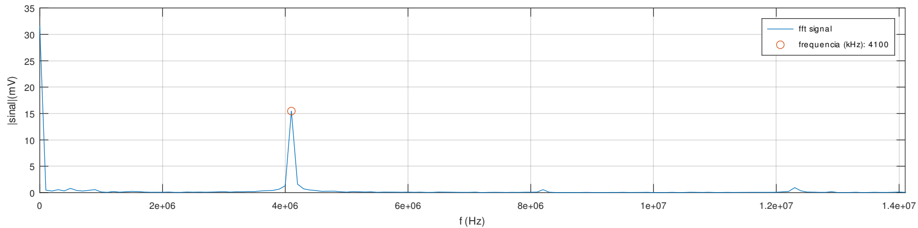
Espectro de amplitudes unilateral X(t) - Saída DC do gerador de sinais com ganho maximo
